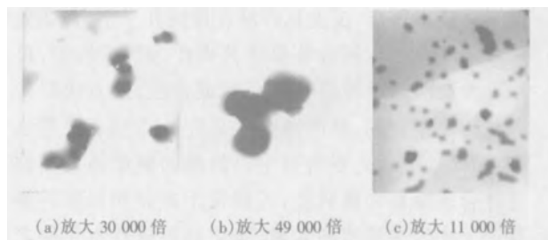
图 3 复合改性乳液的 TEM 照片
