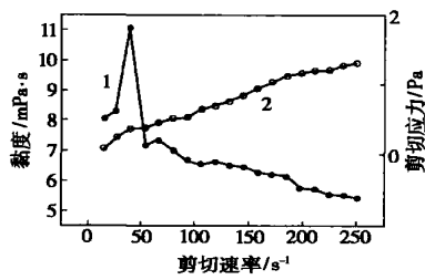
1—黏度;2—剪切应力
