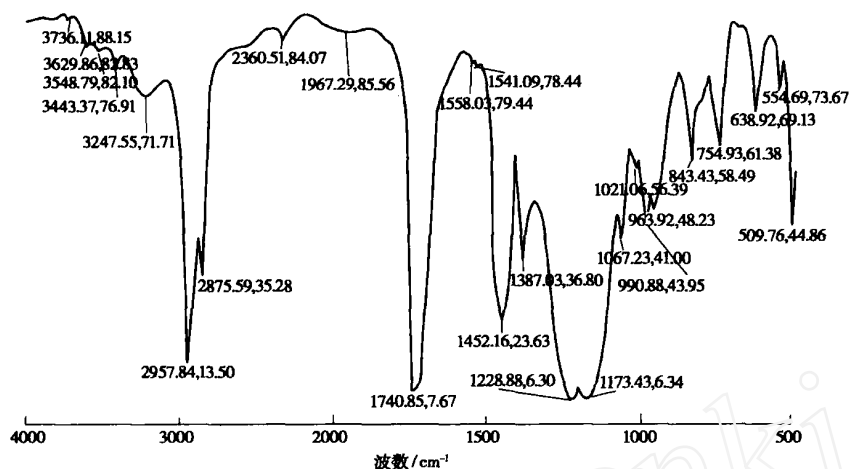
图 1 PTFE-聚丙烯酸酯复合乳液的 FT-IR 谱图
